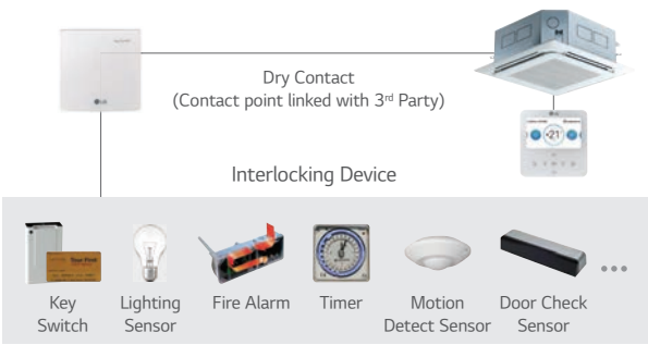
Simple Dry Contact (1 input)
