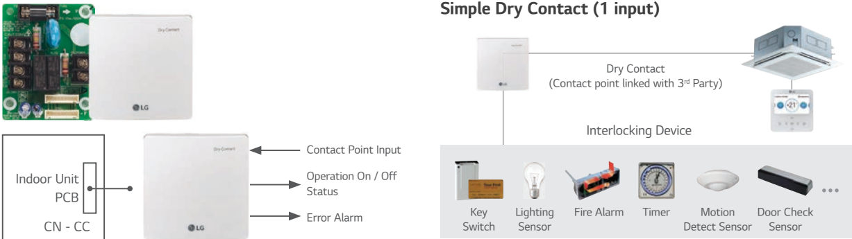
Simple Dry Contact (1 input)
